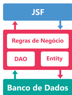
Figura 1: Arquitetura do Sistema.
